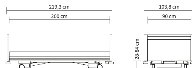
Außenmaße/Höhenverstellbereich:
